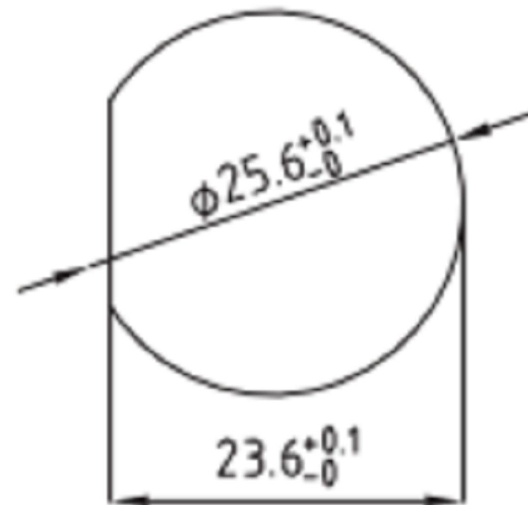
面板开孔尺寸
